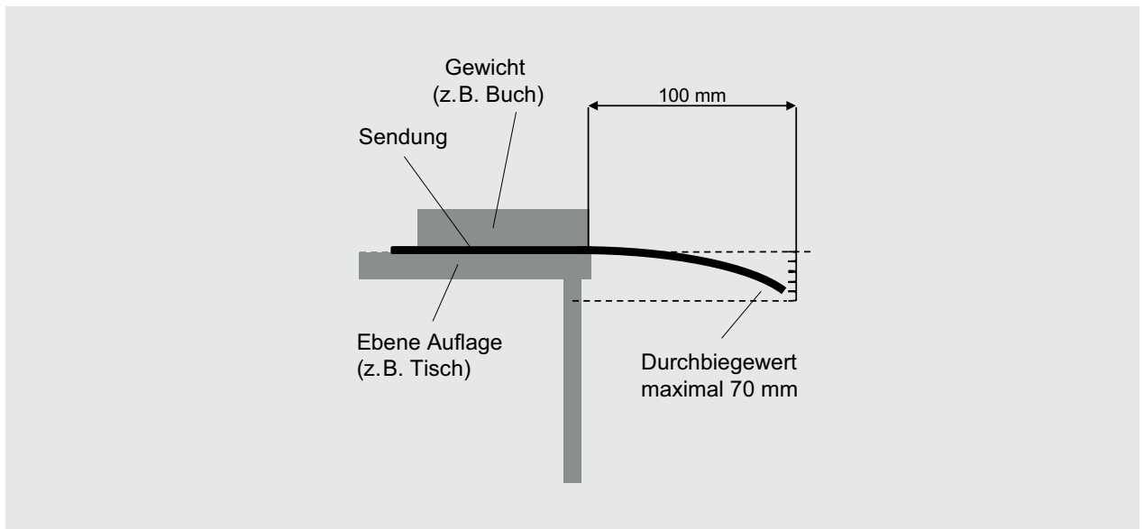
Abb. 31: Schematische Darstellung des Stabilitäts- und Biegefestigkeitstest (Es sind stets alle Ausrichtungen einer Sendung zu prüfen.)
